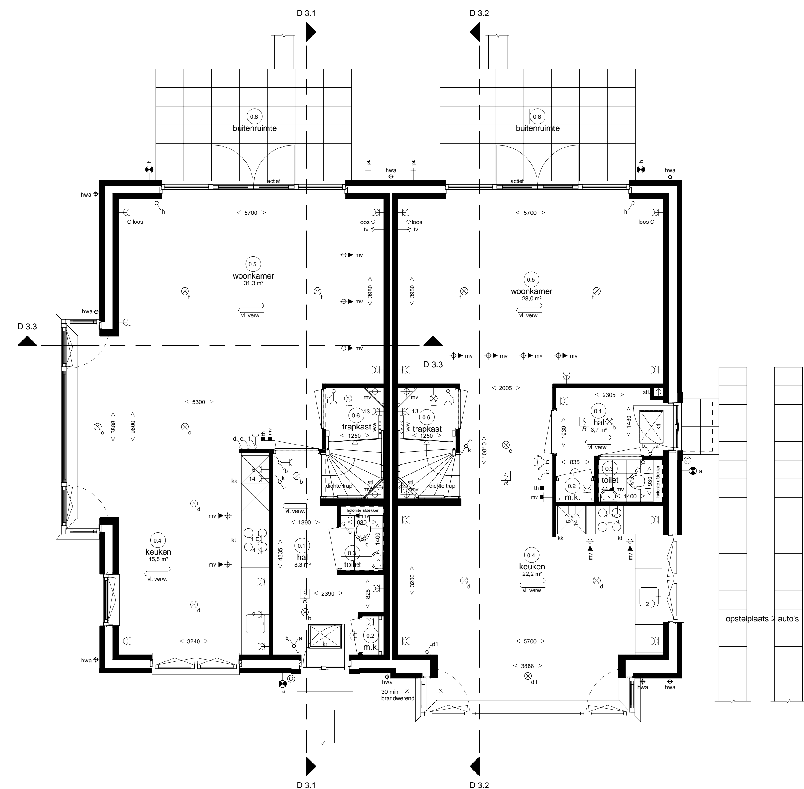
Woningtype B3s Bwnr 38, 46, 54 als get. Bwnr 39, 47, 55 als gesp. Woningtype B4 Bwnr 37, 45, 53 als get. Bwnr 40, 48, 56 als gesp. Begane grond Blok 07, 11, 15 als getekend Blok 08, 12, 16 als gespiegeld
