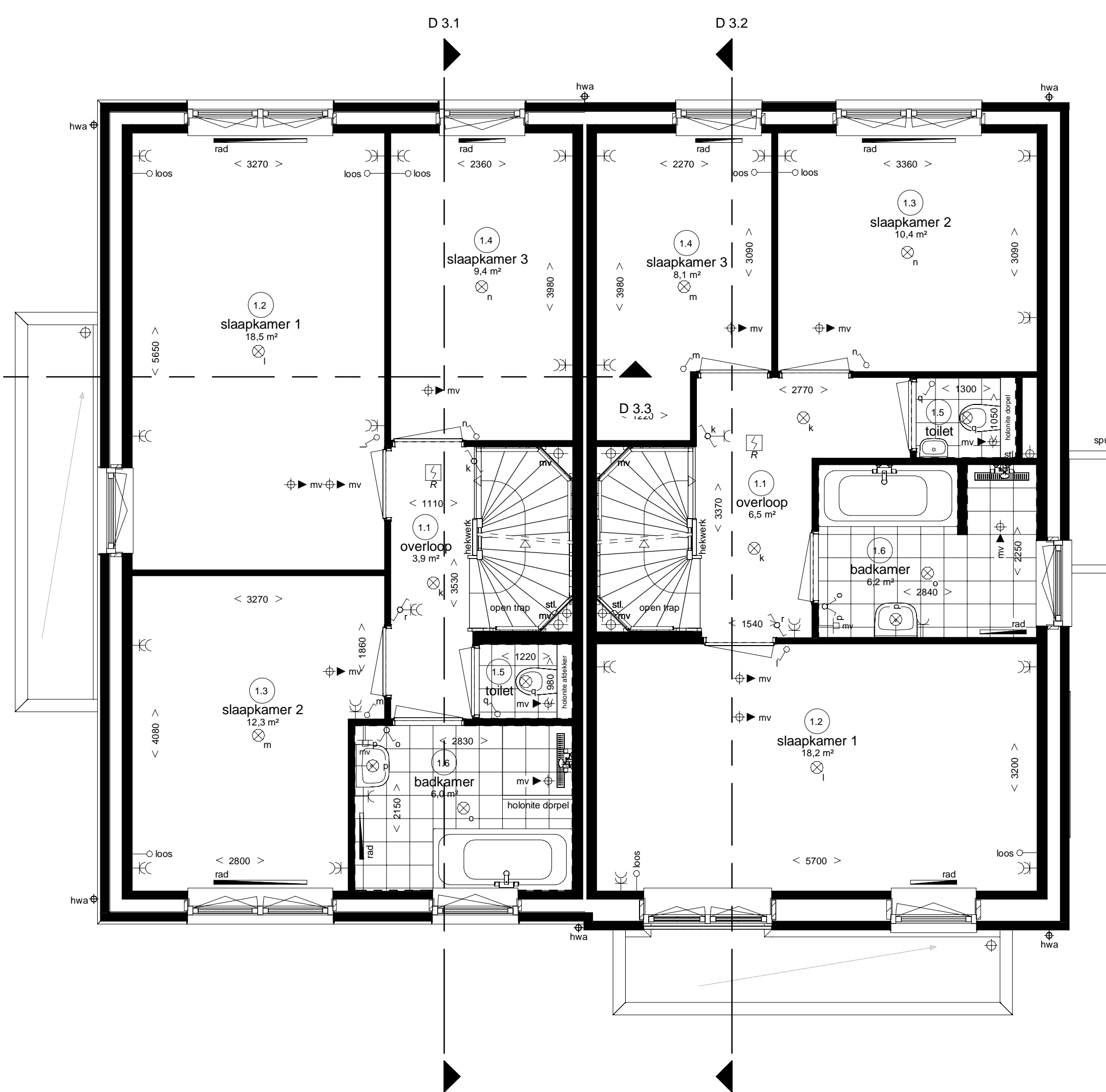
Woningtype B3s Bwnr 38, 46, 54 als get. Bwnr 39, 47, 55 als gesp. Woningtype B4 Bwnr 37, 45, 53 als get. Bwnr 40, 48, 56 als gesp. Eerste verdieping Blok 07, 11, 15 als getekend Blok 08, 12, 16 als gespiegeld
