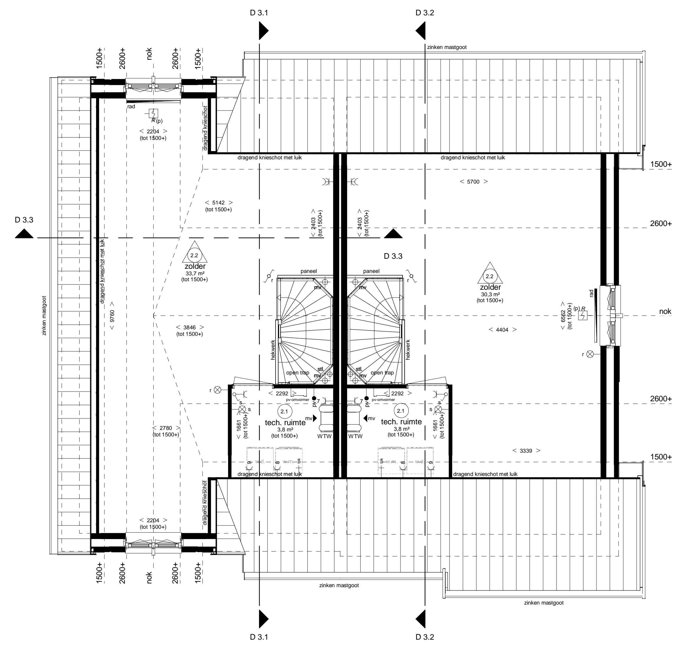
Woningtype B3s Bwnr 38, 46, 54 als get. Bwnr 39, 47, 55 als gesp. Woningtype B4 Bwnr 37, 45, 53 als get. Bwnr 40, 48, 56 als gesp. Tweede verdieping Blok 07, 11, 15 als getekend Blok 08, 12, 16 als gespiegeld
