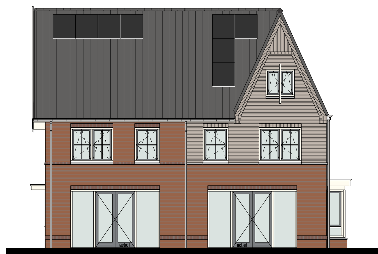
Woningtype B4 Bwnr 40, 48, 56 als gesp. Woningtype B3s Bwnr 39, 47, 55 als gesp.
